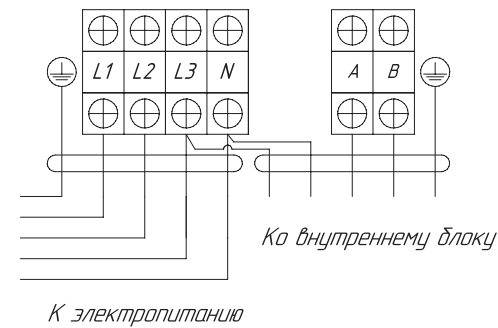
Клеммный терминал наружного блока
