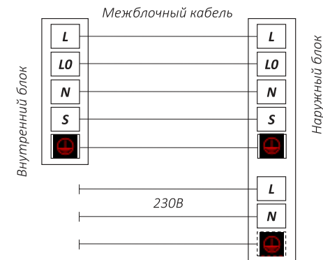
Кабель электропитания* * Кабель электропитания подключен к плате управления наружного блока
